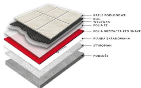
SCHEMAT UŁOŻENIA NA PODŁODZE Z PŁYTKAMI
