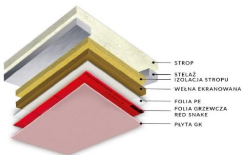
SCHEMAT UŁOŻENIA NA SUFICIE
